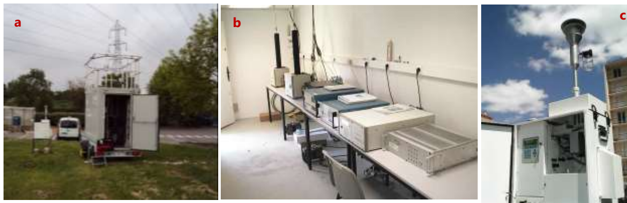
Remorque mobile renfermant les analyseurs installés sur le site de Laurencin (a), exemple d'analyseurs automatiques utilisés pour le NO 2 et PM 10 /PM 2,5 et pour la mesure des métaux (c).
