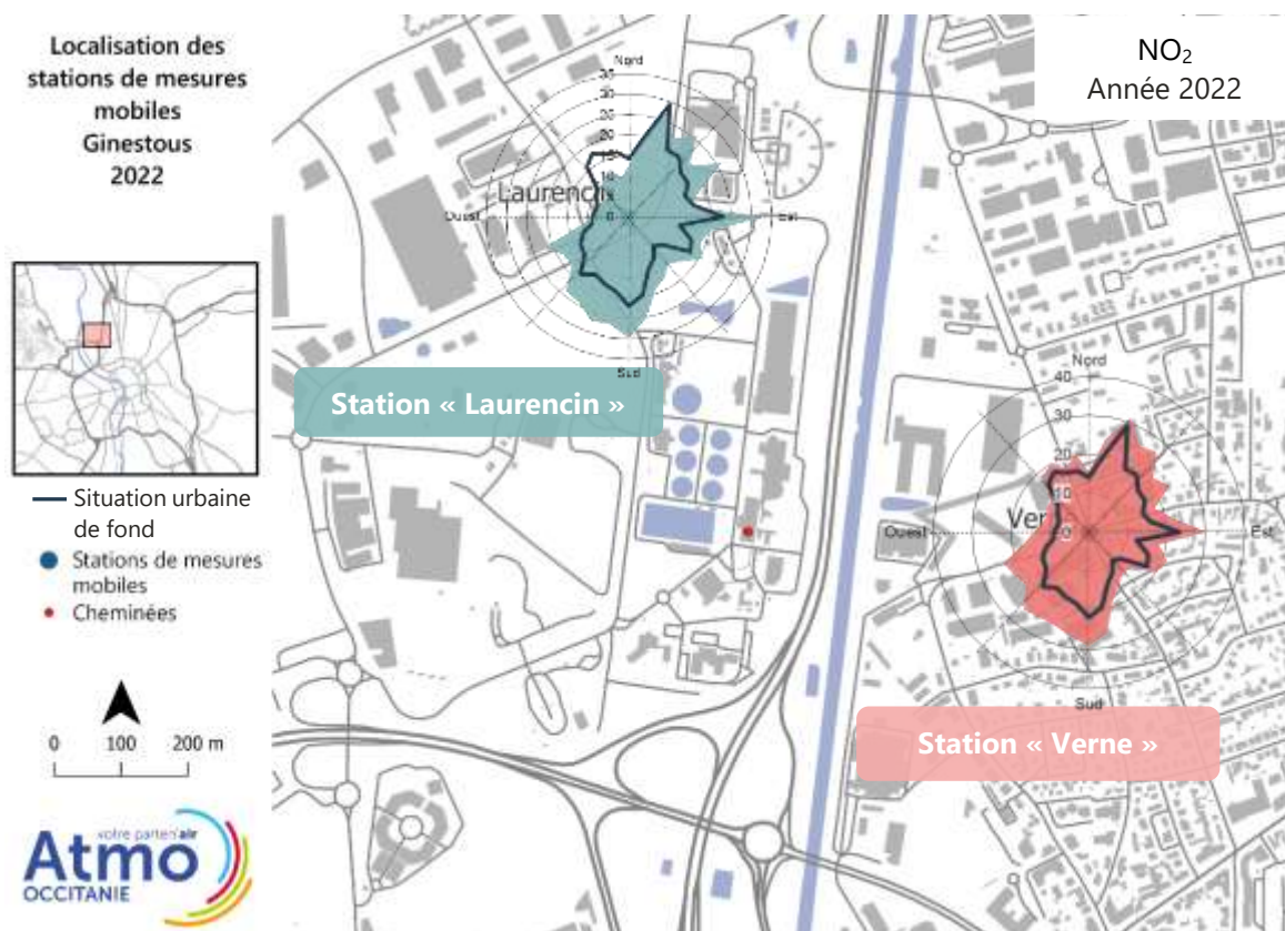
Rose de pollution du dioxyde d'azote (NO 2 ) sur les deux stations "Laurencin" et "Verne".
