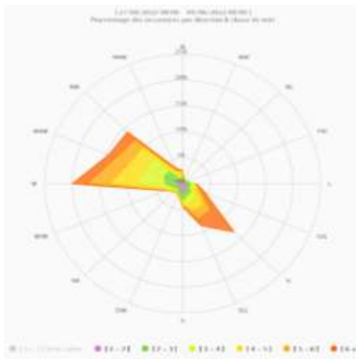
Rose des vents de la station météo Blagnac (Printemps)
