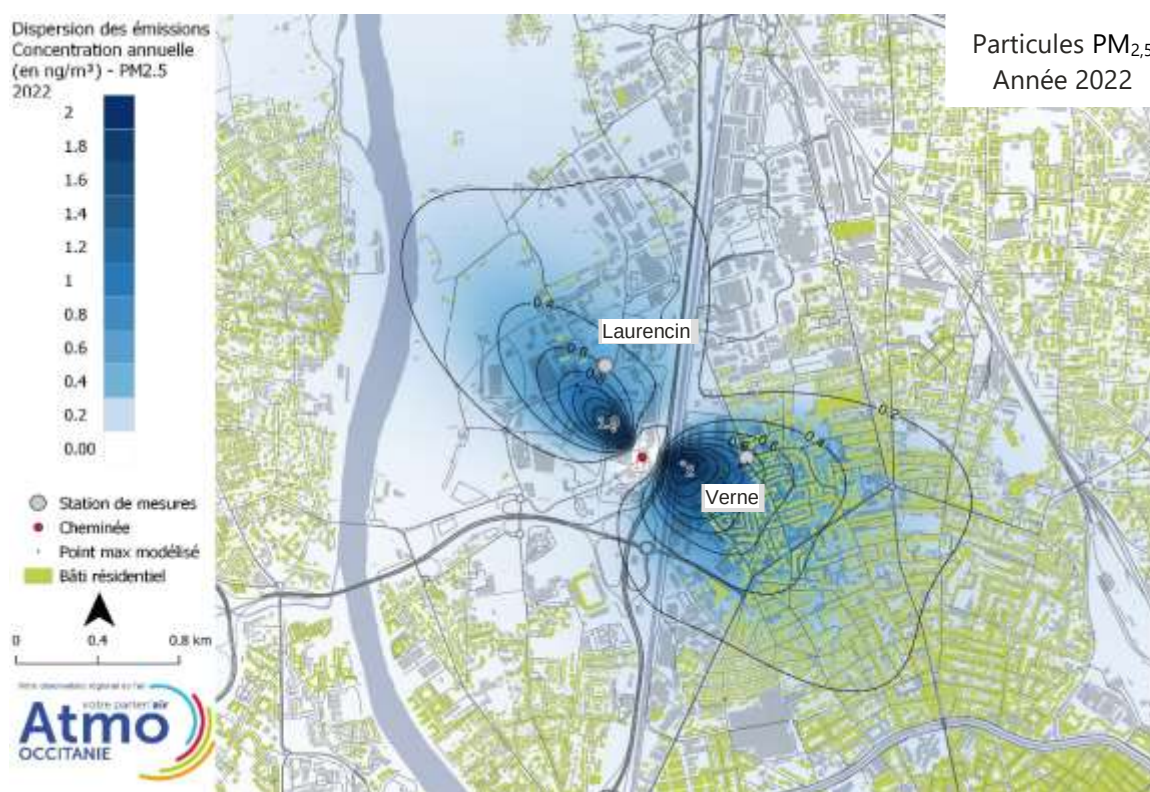
Cartographie de l'impact des rejets de particules PM_{2.5} issues uniquement de l'incinérateur de boues Ginestous-Garonne, sur l'année 2022.
