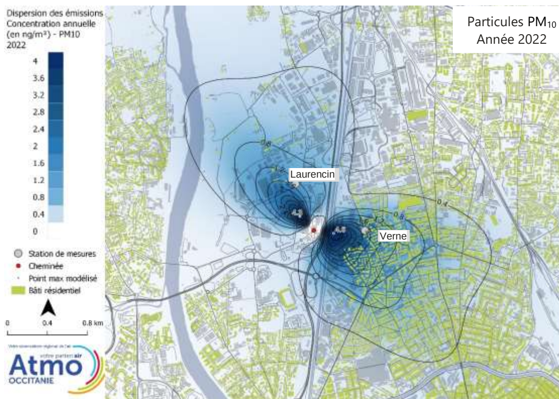
Cartographie de l'impact des rejets de particules PM 10 issues uniquement de l'incinérateur de boues Ginestous-Garonne, sur l'année 2022.
