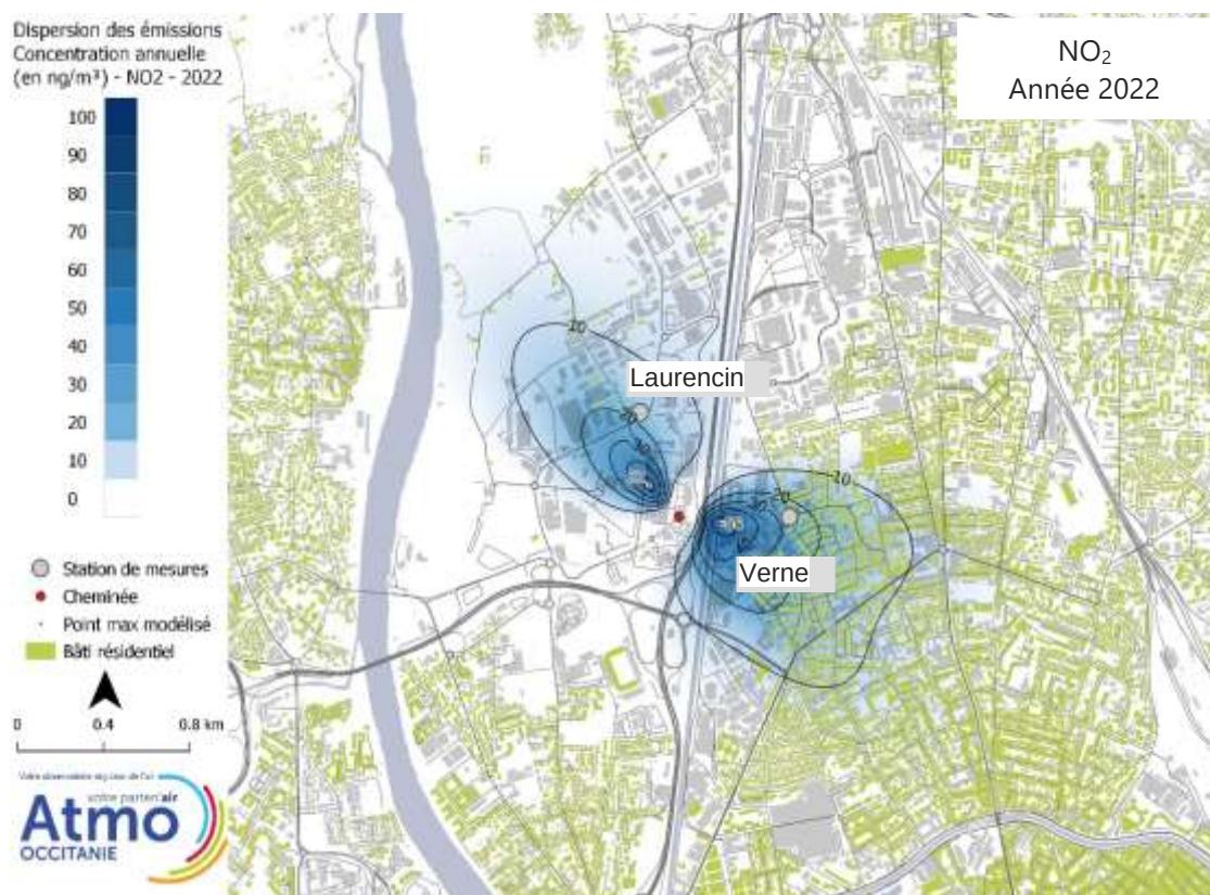
Cartographie de l'impact des rejets de NO 2 issues uniquement de l'incinérateur de boues Ginestous-Garonne, sur l'année 2022.
