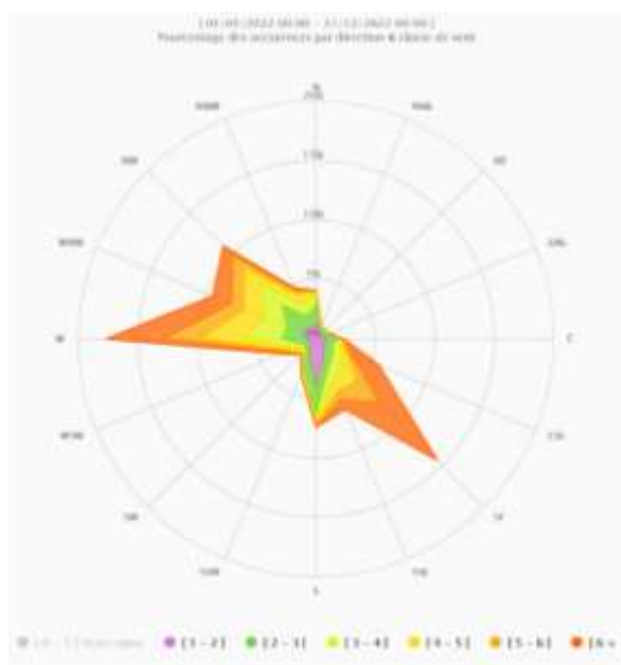
Rose des vents de la station météo Blagnac (Année 2022)
